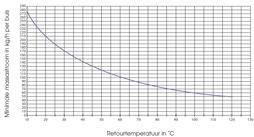
Relatie tussen minimale massastroom en retourtemperatuur
